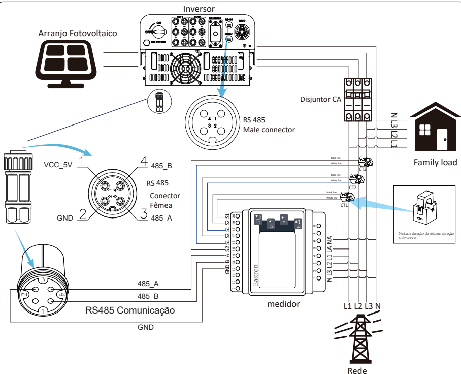
Figura 14 Diagrama da Comunicação do medidor Eastron
