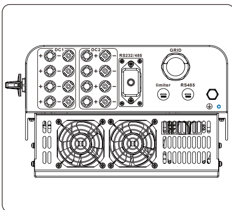
Fig 1.2 Vista Inferior
