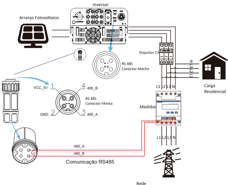
Figura 7.16 Conexão do diagrama do medidor CHINT
