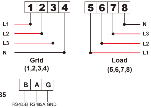
Figura 7.11 Medidor Eastron
